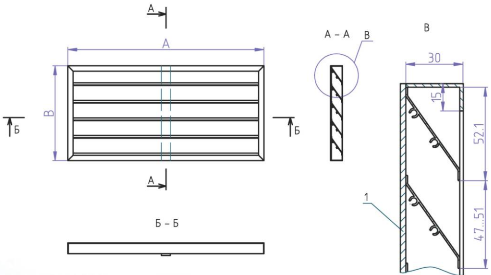
Наружная накладная решётка OGW AxB (габаритный размер решётки)
